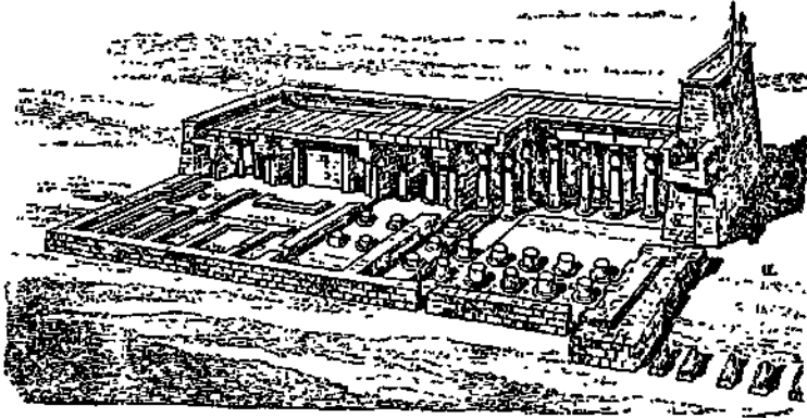
شكل ١٢٦ - رسم هندسى يمثل تفاصيل المعابد ذات الصروح في عهد الامبراطورية . وقد روى رسم نصف المعبد ونصف الصرح المقابل للقائى لانهما يحتويان المعبد (ماخوذ عن برو وشييه)
